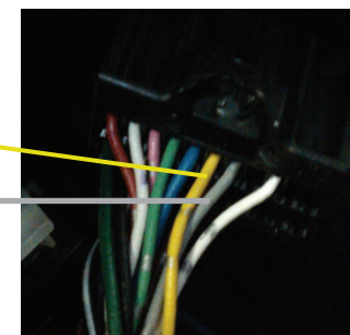
Fio Amarelo casa 6 Fio Cinza casa 7
