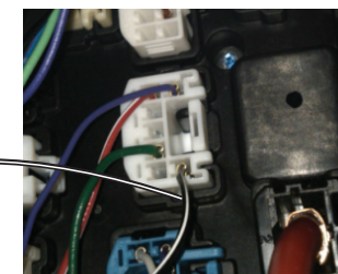
Fio Preto/Branco sinal das portas
