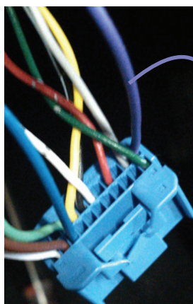
Fio roxo, pós chave (coluna esquerda)
